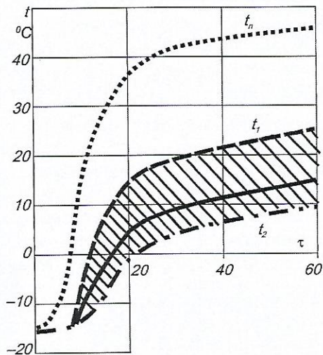
Rysunek 13.18. Wykresy temperatury nagrzewania kabiny ciągnika z nagrzewnicą A przy temperaturze otoczenia -15^{\circ}\text{C} :
