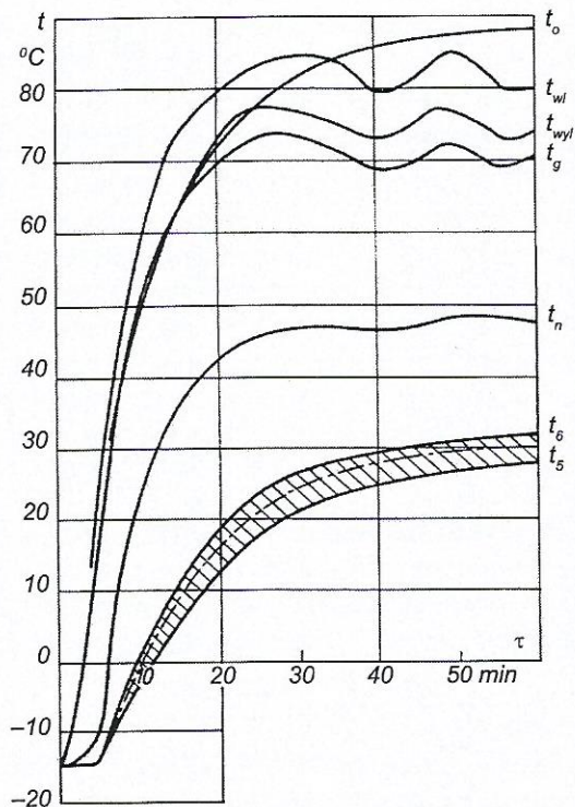
Rysunek 13.19. Wykresy temperatury nagrzewania kabiny ciągnika z nagrzewnicą B przy temperaturze otoczenia -15^{\circ}\text{C} :
